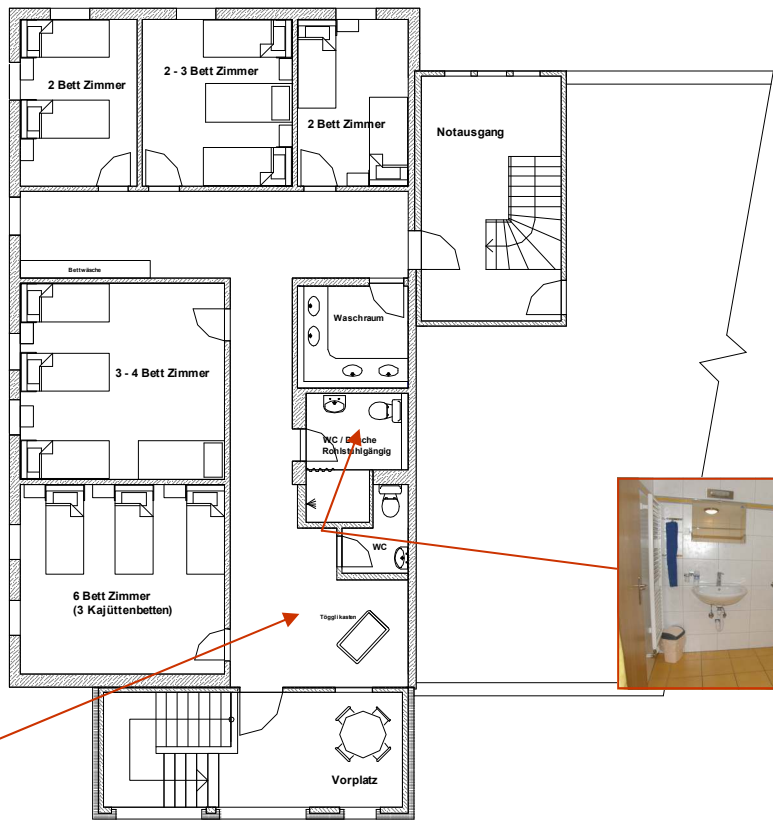
Grundriss OG
